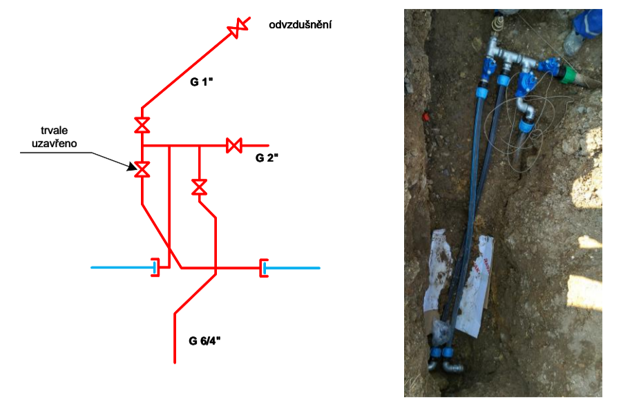
DETAIL Y
